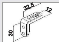
Uchwyt żyłki kątowy
